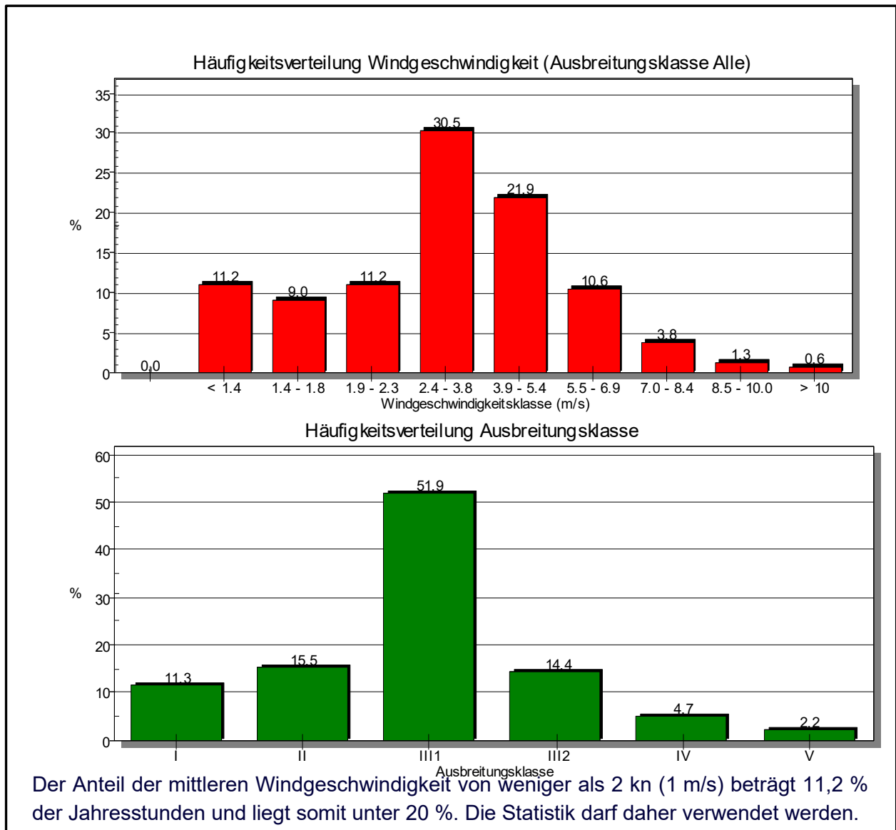
Abbildung 3: Windgeschwindigkeit und Ausbreitungsklassen der Station Oldenburg. Zeitraum: 1998 bis 2007
